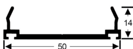
MC-878 | 0,397 kg/m
