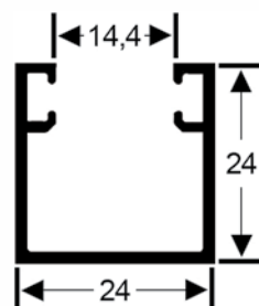
MC-6 | 0,304 kg/m
