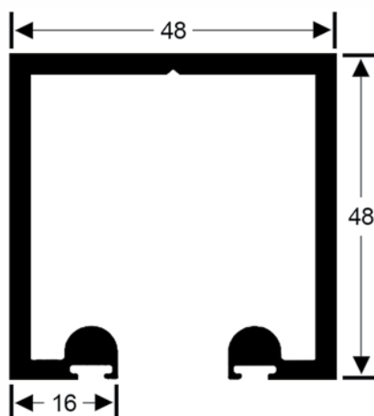
MC-68 | 1,366 kg/m
