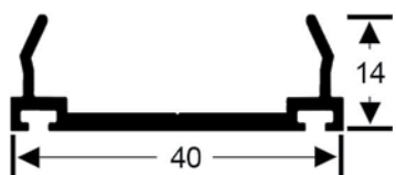
MC-615 | 0,344 kg/m
