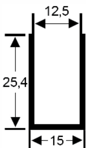
MC-10 | 0,209 kg/m
