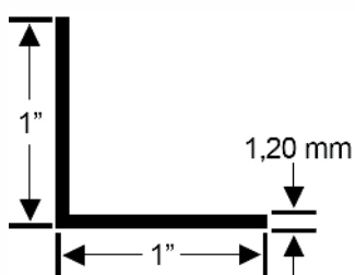
MC-90 | 0,166 kg/m
