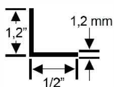
MC-92 | 0,083 kg/m
