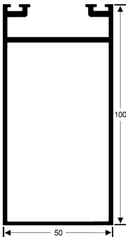
MC-96 | 2,004 kg/m
