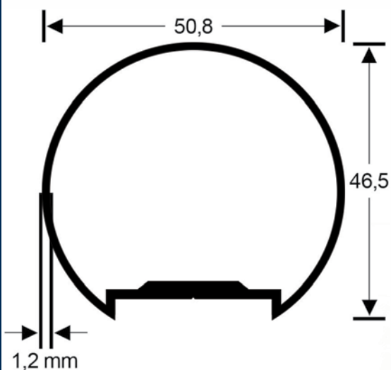
MC-333 | 0,628 kg/m
