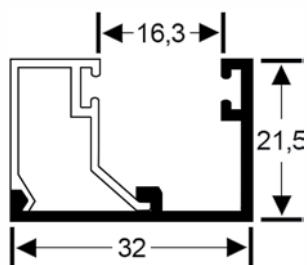
MC-26 | 0,253 kg/m
